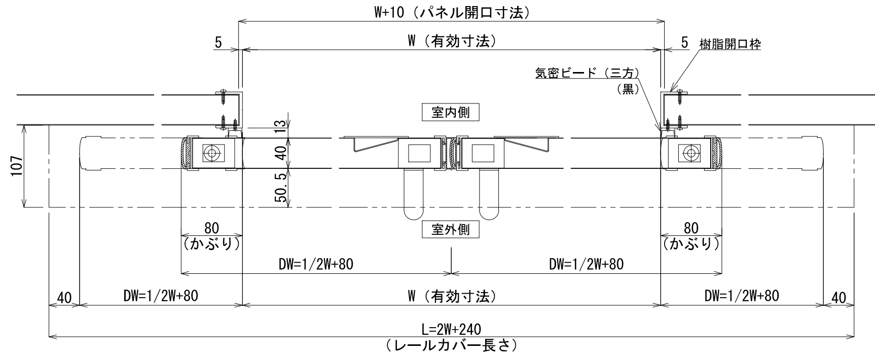
正面図 S=1/30
