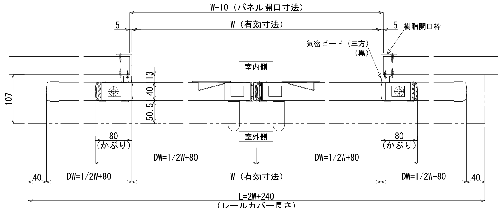
横断面図 S=1/5
