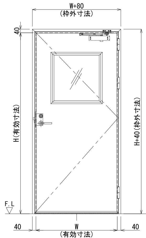
正面図 S=1/20
