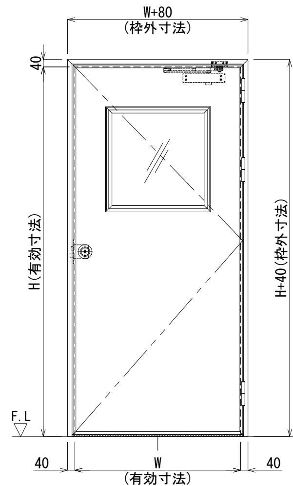
正面図 S=1/20
