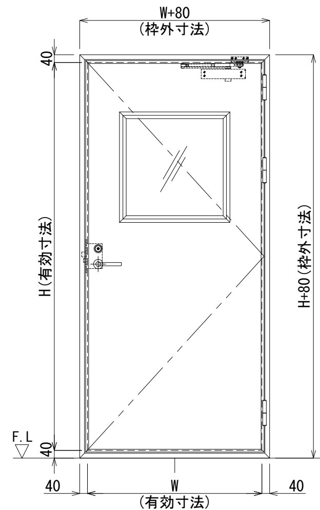
正面图 S=1/20
