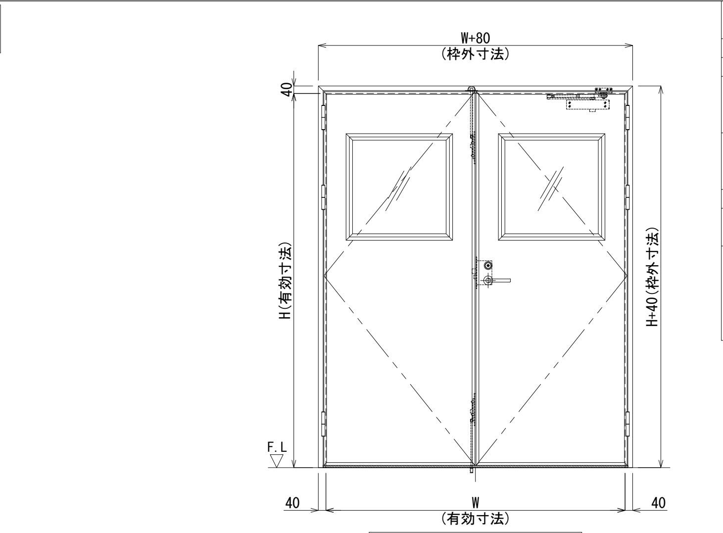
正面図 S=1/20 ※この姿図は右親を表す
