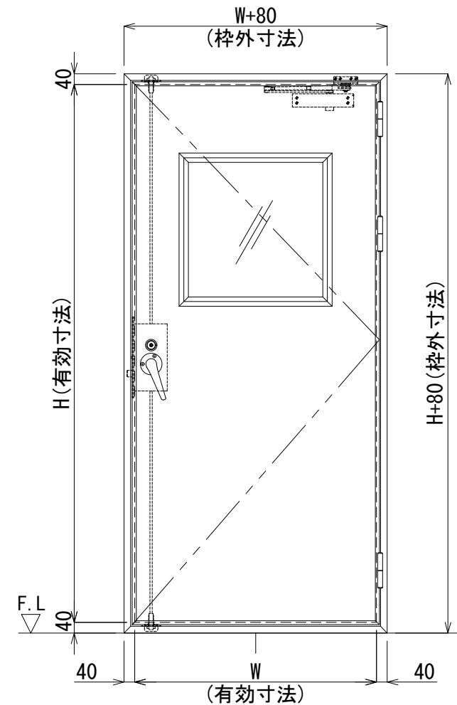
正面图 S=1/20
