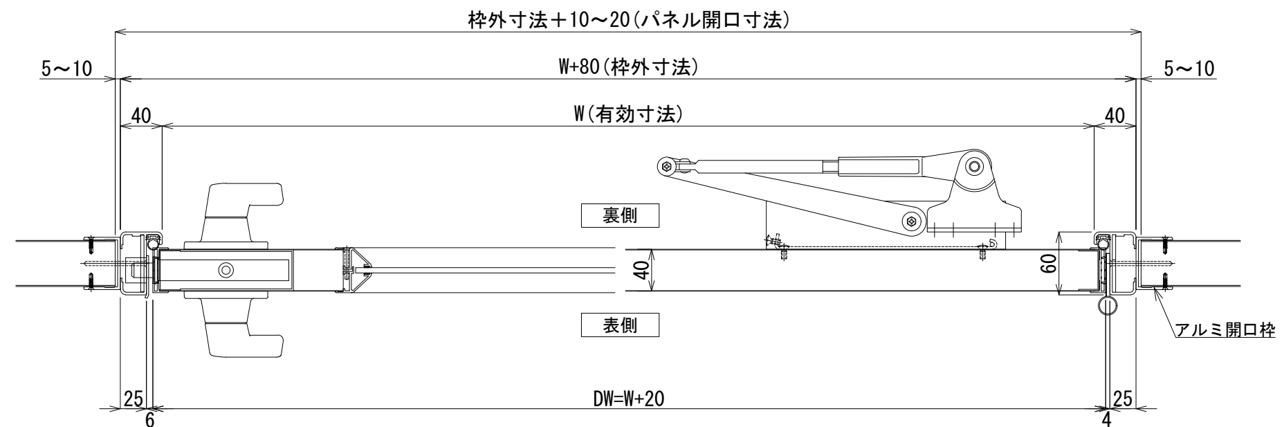
横断面図 S=1/5
