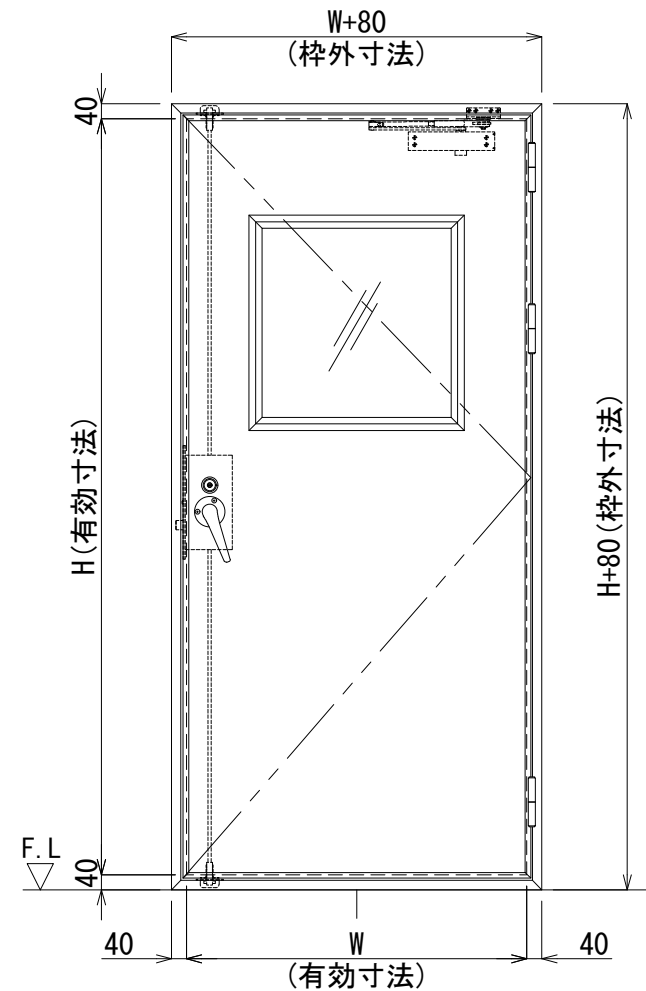
正面図 S=1/20
