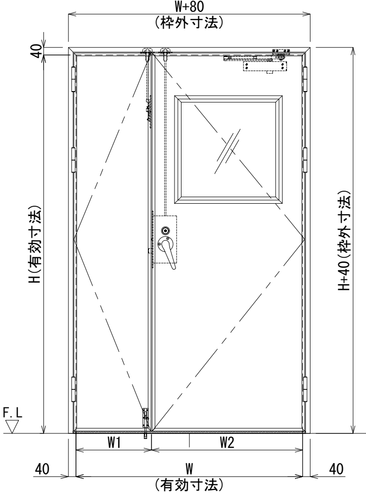
正面図 S=1/20
