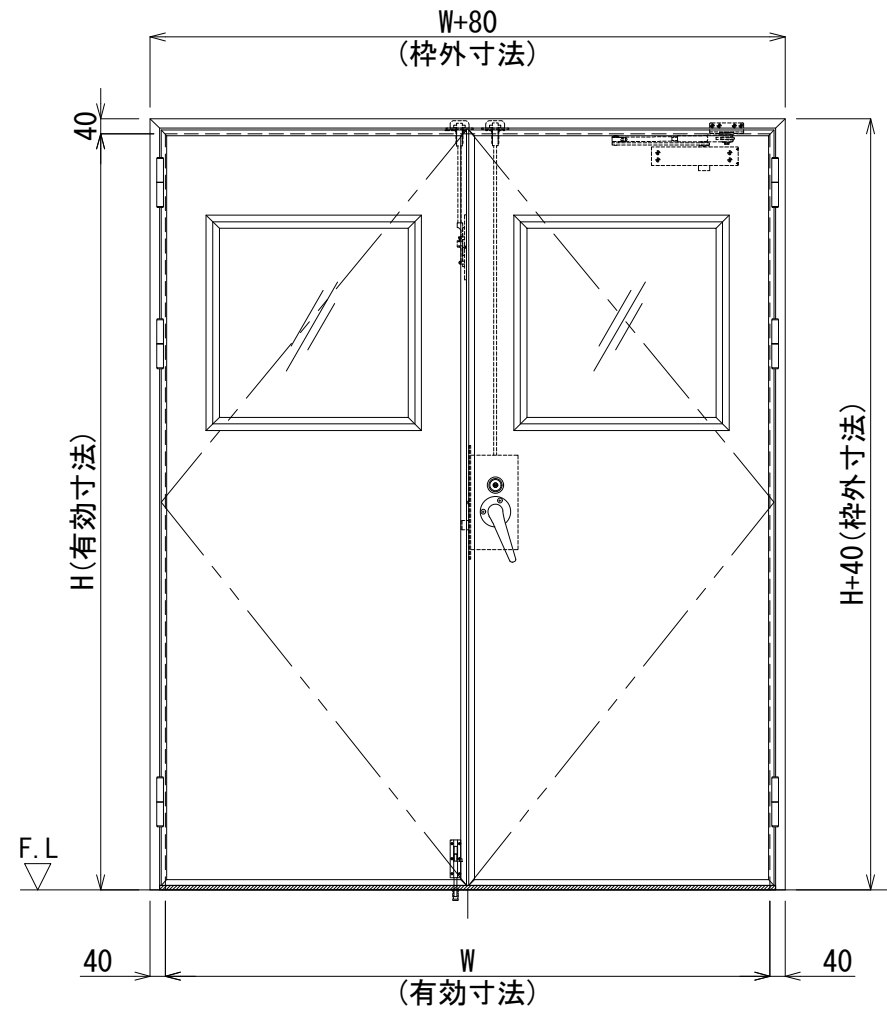
正面図 S=1/20 ※この姿図は右親を表す
