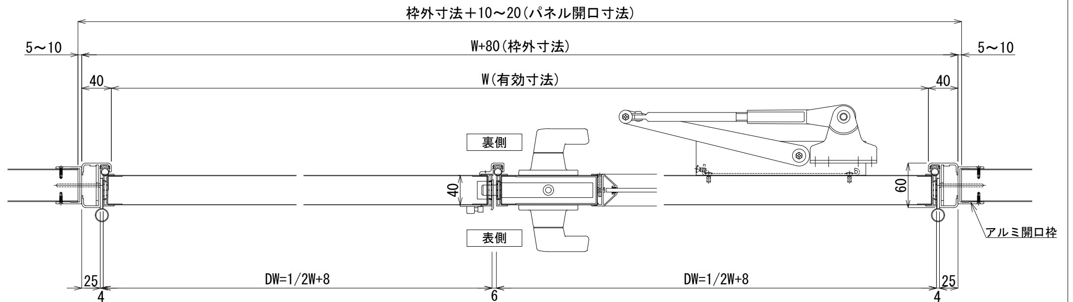
横断面図 S=1/5 ※この図は右親を表す
