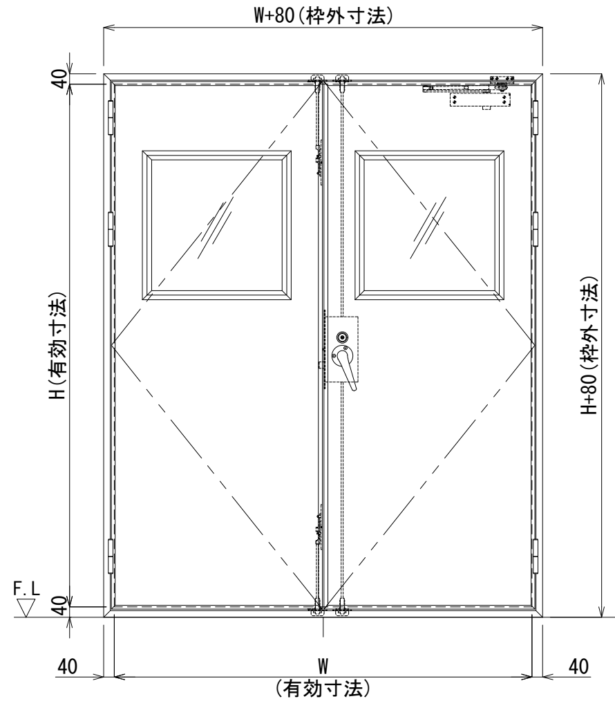
正面図 S=1/20
