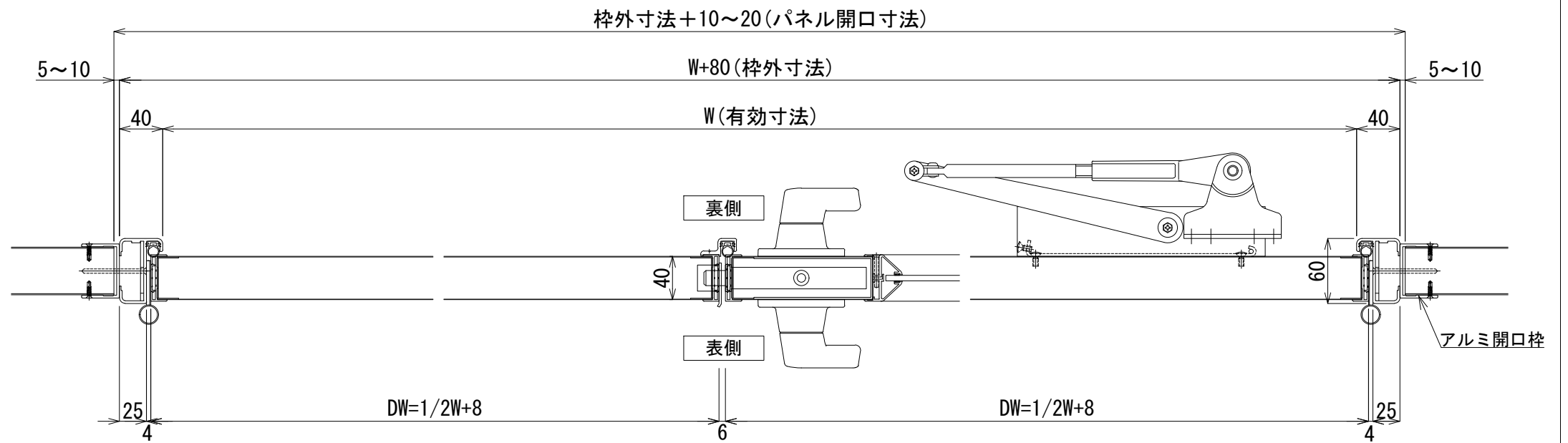
横断面図 S=1/5
