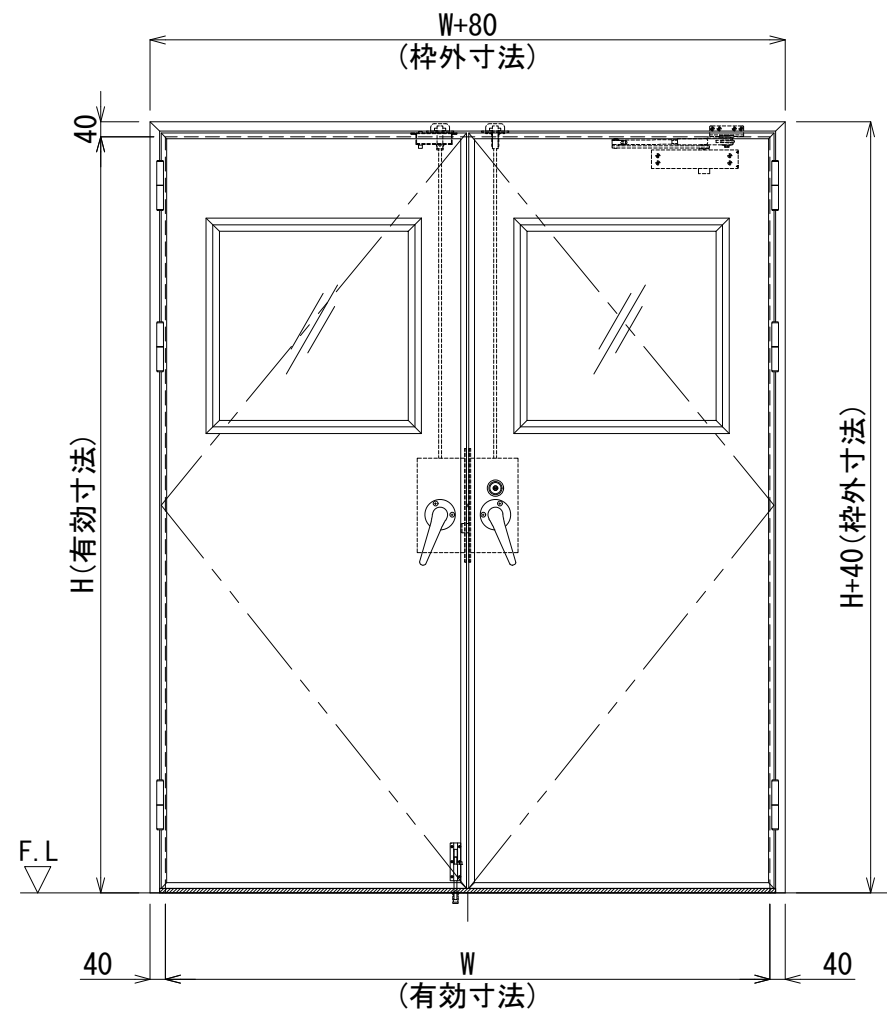
正面図 S=1/20
