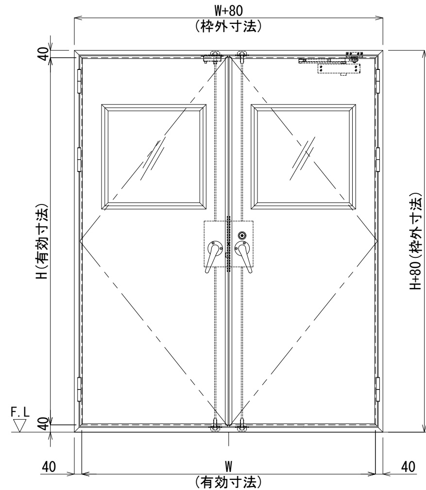
正面図 S=1/20 ※この姿図は右親を表す
