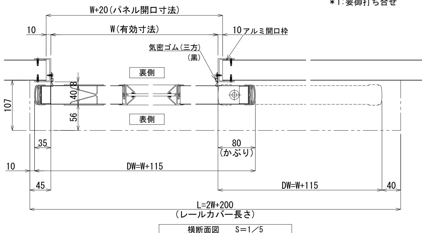
正面図 S=1/30 ※この姿図は右引を表す
