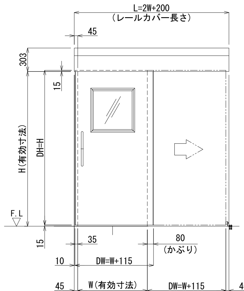
正面图 S=1/30
