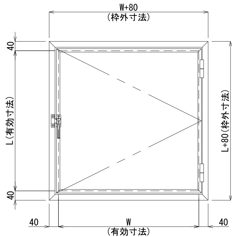
【 庫内開き 】
