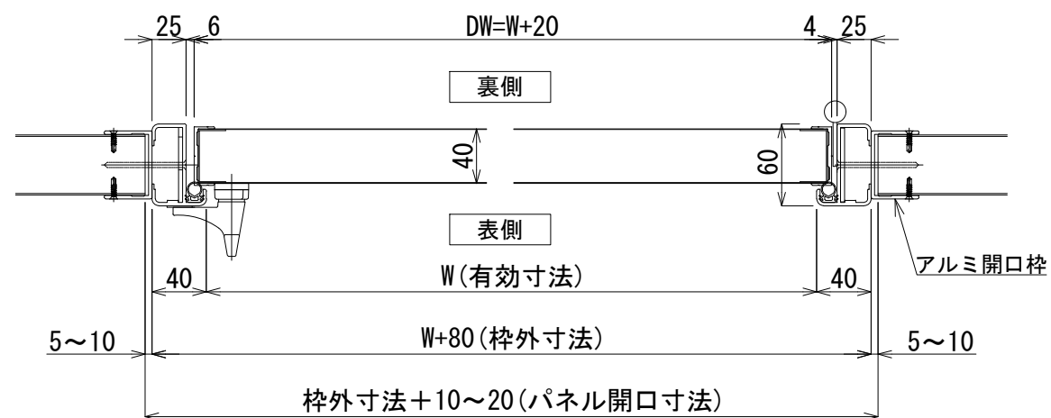
【 庫外開き 】
