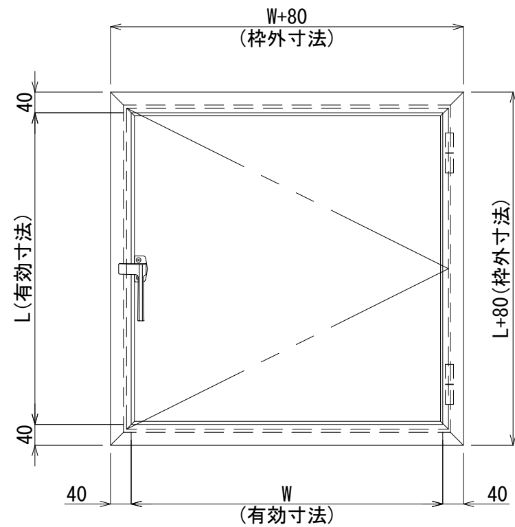
【 庫外開き 】
