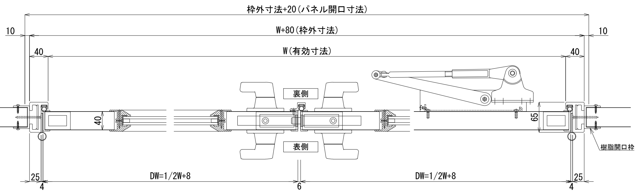
横断面図 S=1/5 ※この図は右親を表す
