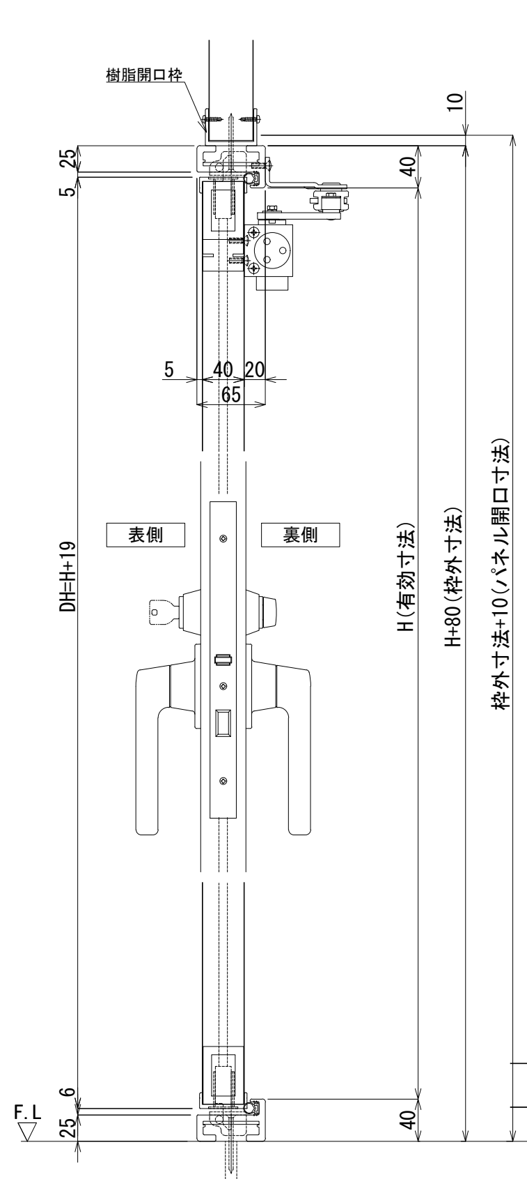
縦断面図 S=1/5
